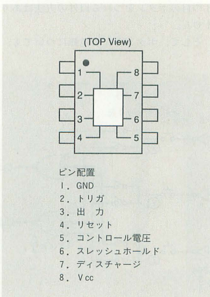
図3 555端子表
